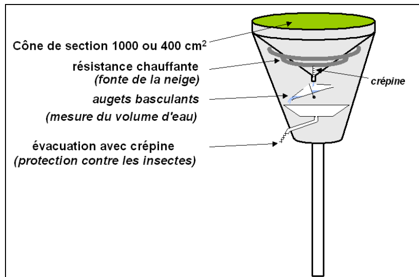
Figure 2 : Schéma d'un pluviomètre © Météo-France, extrait de cours de l'École Nationale de la Météorologie (ENM)
