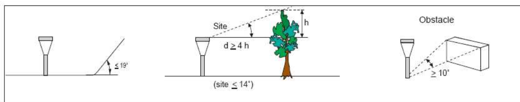
Figure 8 : Schéma illustrant la classe 1 du pluviomètre (installation idéale)
